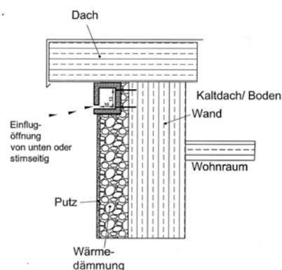
Hinterdämmtter Einbaustein
