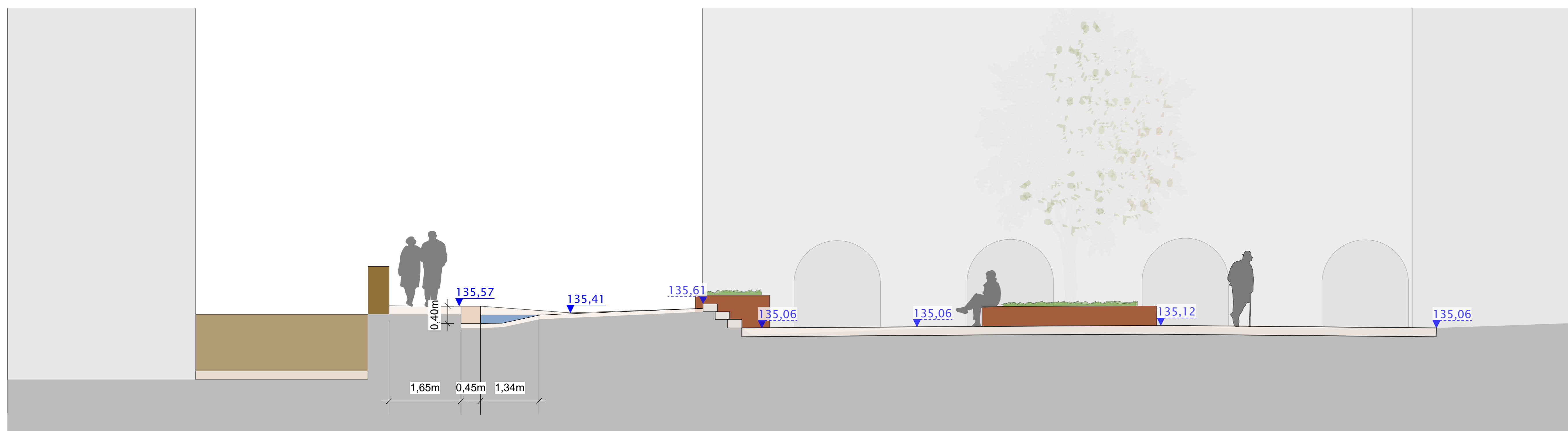
Schemaschnitt – Rheinpfalz
